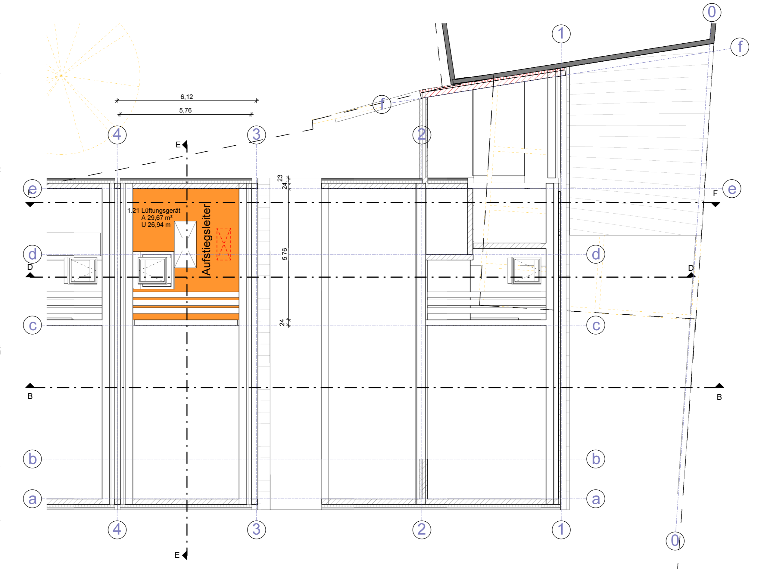
Grundriss Dachgeschoss - M 1:100
